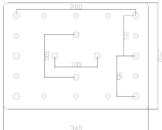
Grundplatte
